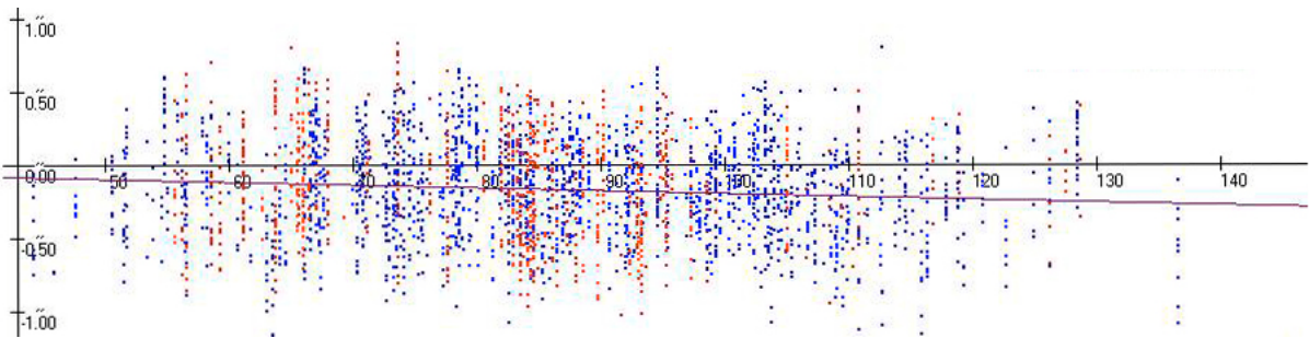
График 2. Распределение остаточных разностей (O-C) по склонению Венеры в зависимости от значения фазовых углов.
