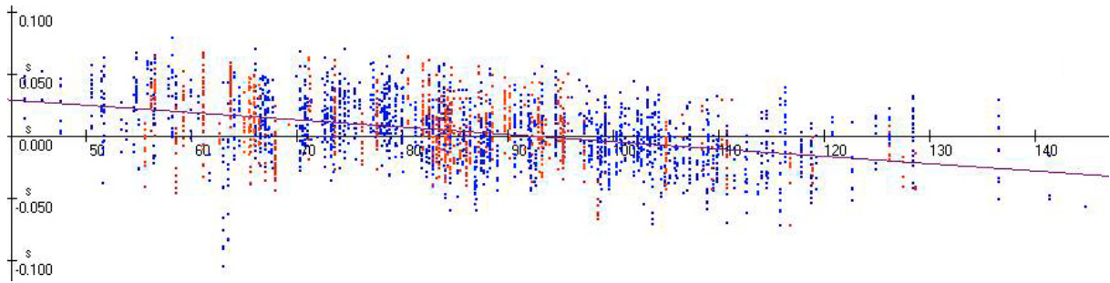
График 1. Распределение остаточных разностей (O-C) по прямому восхождению Венеры в зависимости от значения фазовых углов.
